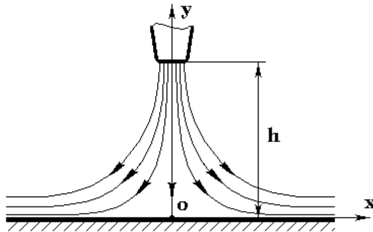
Схема натекания потока газа из сопла горелки на плоскость
