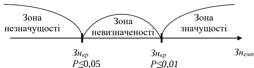
Рис. 1. Графічна схема визначення значущості статистичного критерію.
