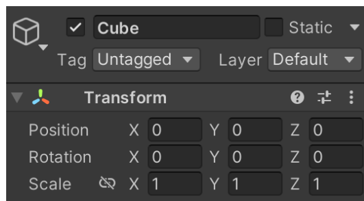
Рисунок 2.4 – Компонент Transform
