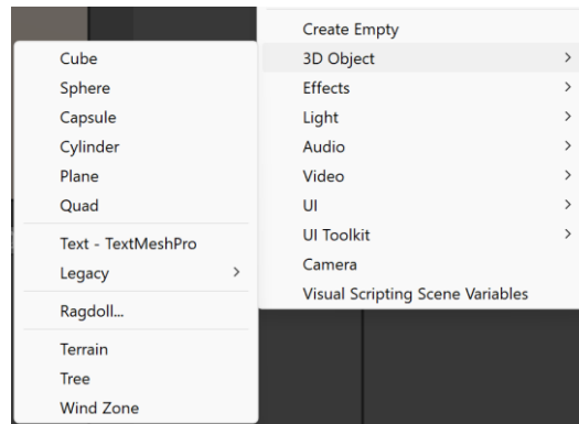
Рисунок 2.2 – Приклад GameObject
