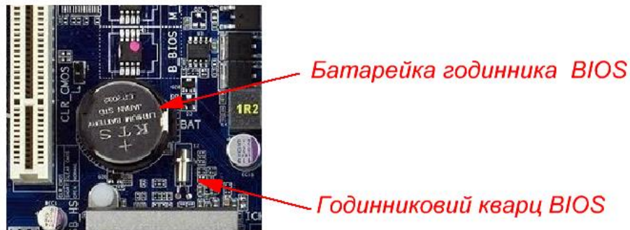
Рисунок 6 – Годинниковий кварц на материнській платі комп'ютера
