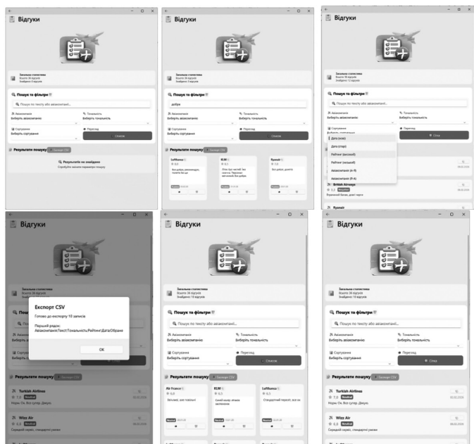
Рис. 1. Перегляд відгуків з фільтрацією у режимі сітка/список
