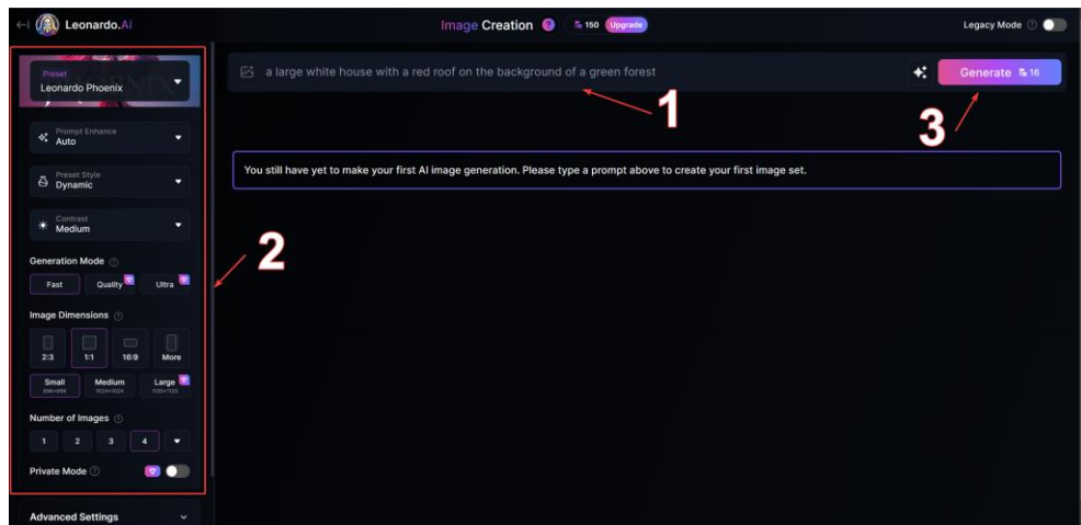
Рисунок 2.8 – Порядок роботи з системою Leonardo.Ai
