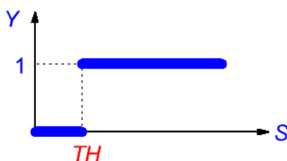
Рисунок 6.3 – Порогова активаційна функція
