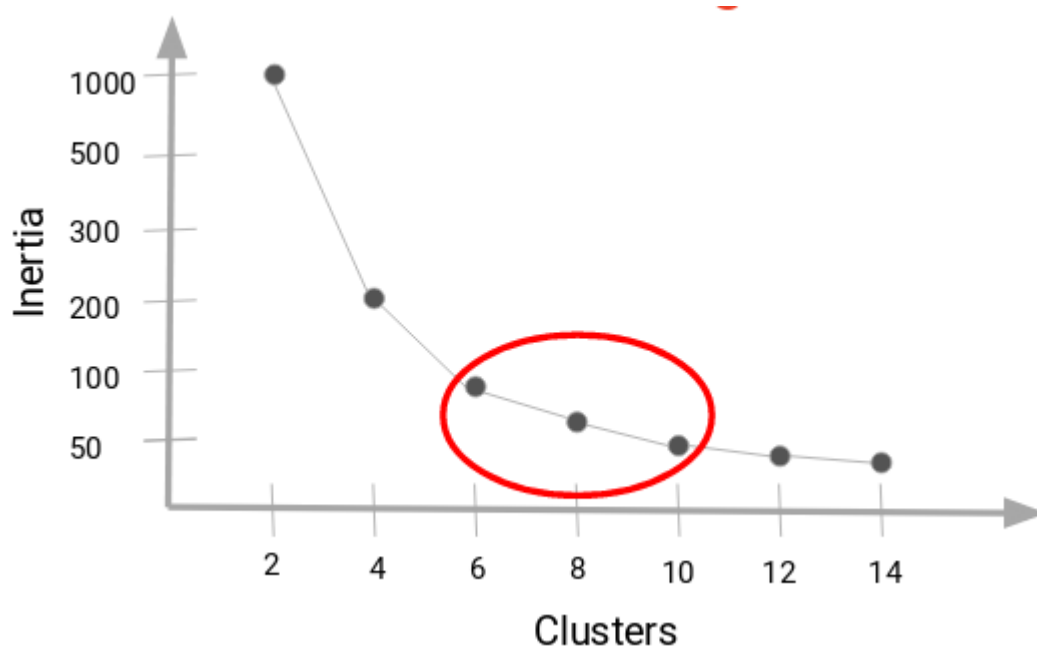
Рисунок 4.4 – Крива ліктя, де у якості метрики обрана інерція
