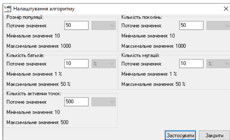
Рисунок 8.4 – Налаштування параметрів генетичного алгоритму
