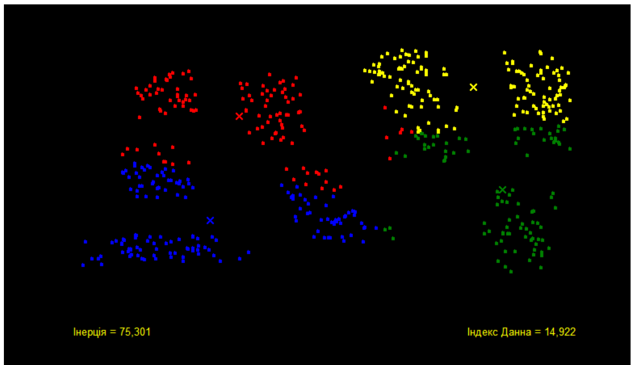
Рисунок 4.13 – Процес кластеризації
