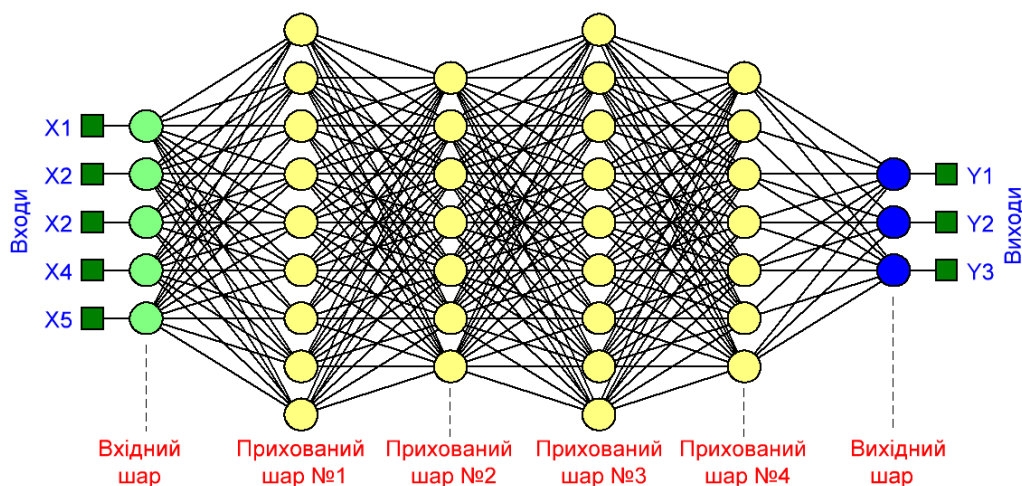
Рисунок 6.4 – Нейронна мережа
