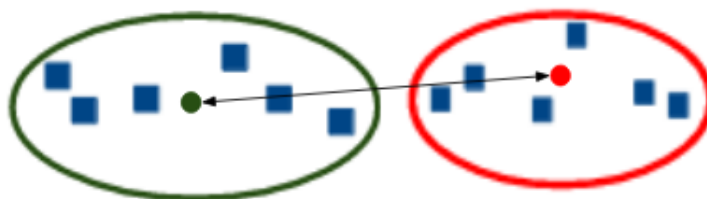
Рисунок 4.3 – Міжкластерна відстань
