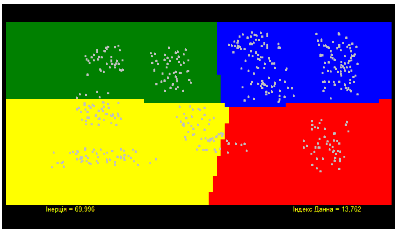
Рисунок 4.14 – Результат кластеризації
