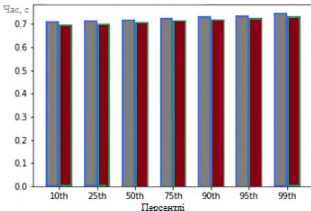
Рисунок 3.6 – Результати тестування CodeGuida, прапор компілятора O2
