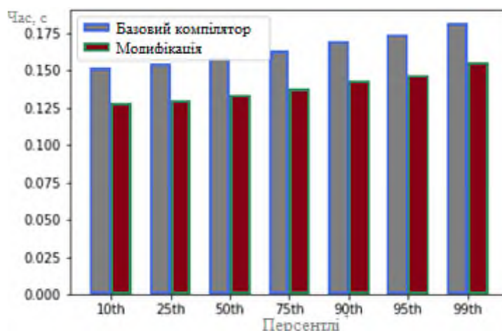
Рисунок 3.9 – Результати тестування Cartesian Tree, прапор компілятора O2
