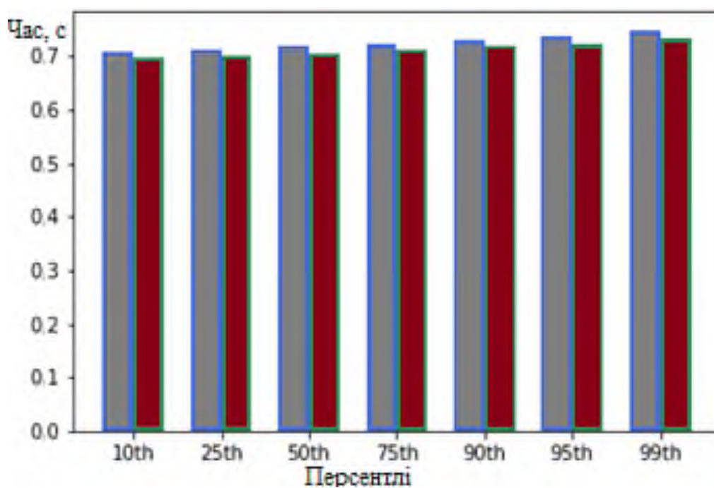
Рисунок 3.7 – Результати тестування CodeGuida, прапор компілятора O3
