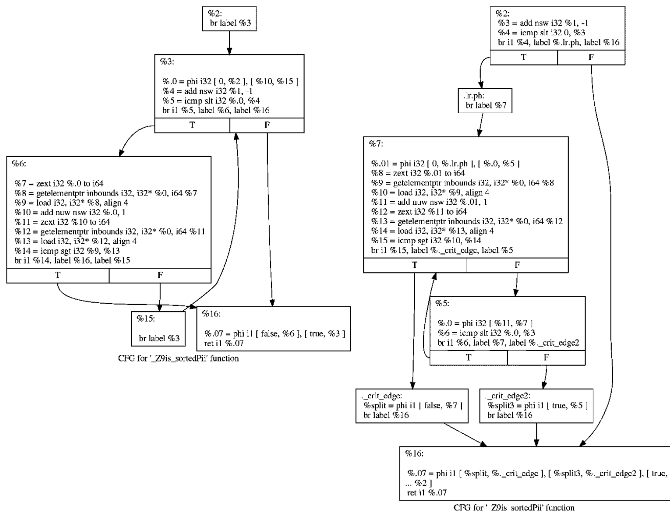
Рисунок 2.1 – Графік передачі управління до і після проходу ротації циклів
