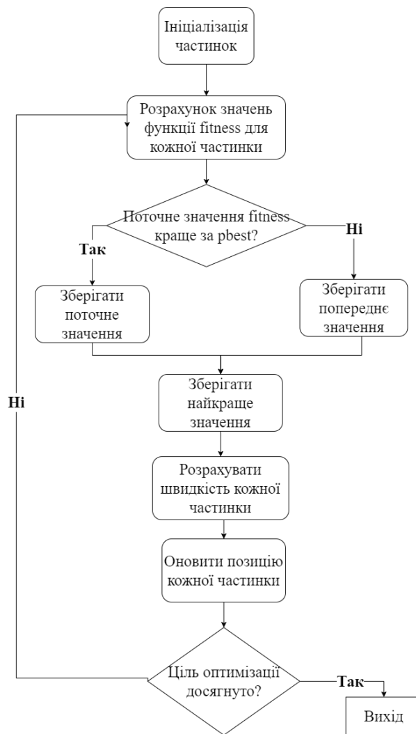
Рисунок 2. Алгоритм рою частинок
