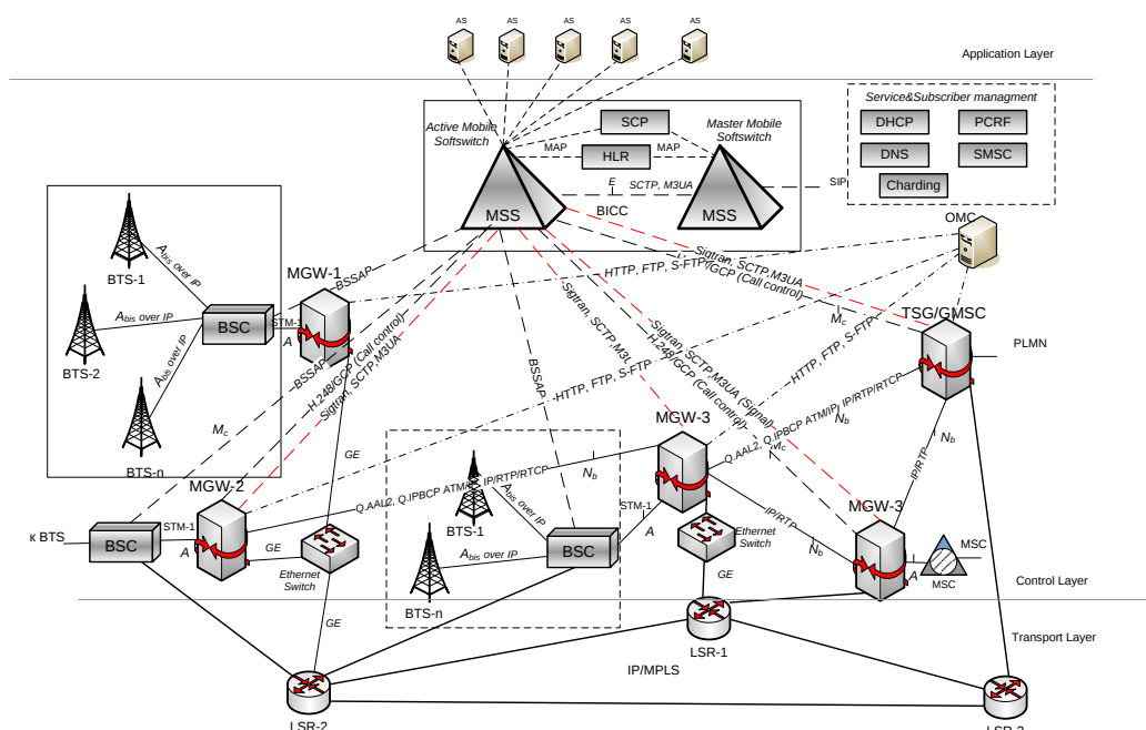
Рисунок 3 – Мережа мобільного зв'язку, побудована на базі медіашлюзів MGW
