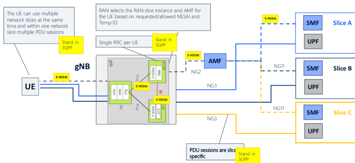
Рисунок 10 – Віртуалізація Network Slicing [11]
