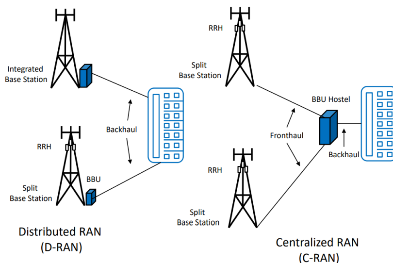
Рисунок 6 – Реалізація C-RAN та D-RAN
