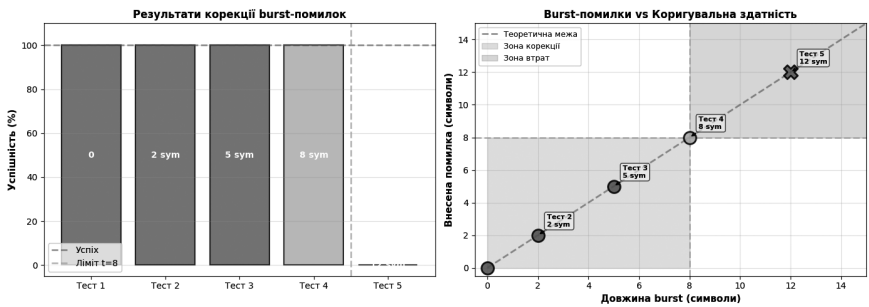
Рис. 1. Результати корекції burst-помилки
