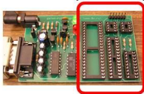
Програматор (мікроконтролер встановлюється у спеціальні панельки)
