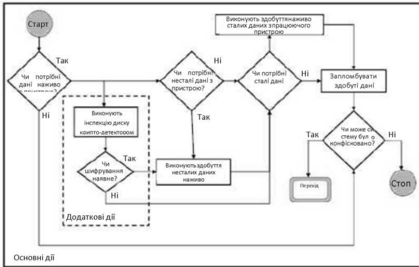
Рис. 3. Настанови для здобуття потенційних цифрових доказів на увімкнених цифрових пристроях
