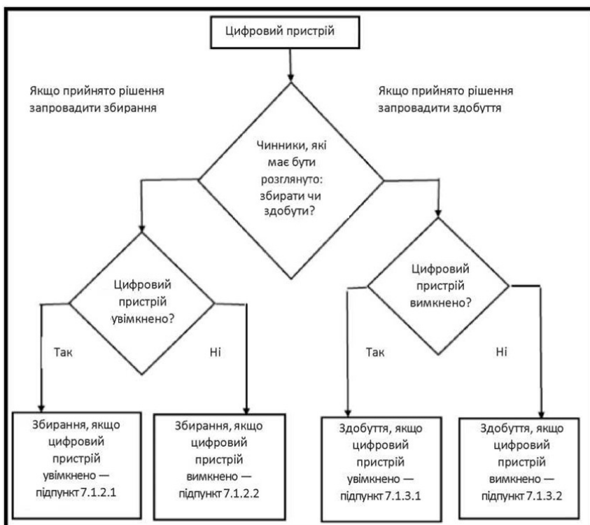
Рис. 1. Настанова для процесу прийняття рішення збирати чи здобути потенційні цифрові докази
