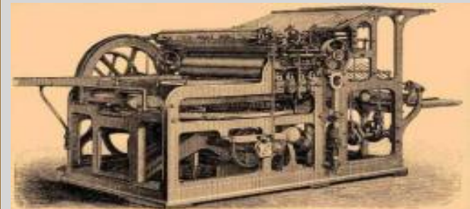
1. Парова швидкодрукувальна машина «Політех» в Вюрттемберзі.
