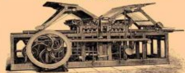
3. Парова швидкодрукувальна машина «Політех» в Вюрттемберзі.
