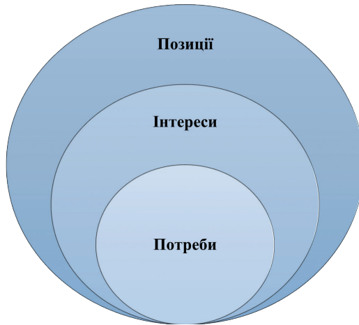
Рис. 2. Позиції–інтереси–потреби
